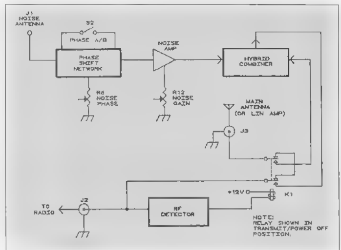
Figuur 1: Hier blijkt hoe simpel de schakeling is: een regelbaar faseverschuivingsnetwerk waarmee de storing precies 180 graden in fase kan worden verschoven. De daarachter geplaatste versterker en de combiner waarin de signalen weer gemengd worden. De RF-detector kijkt of er zendenergie aanwezig is, om zo het relais af te kunnen laten vallen en zodoende het apparaat te overbruggen.
